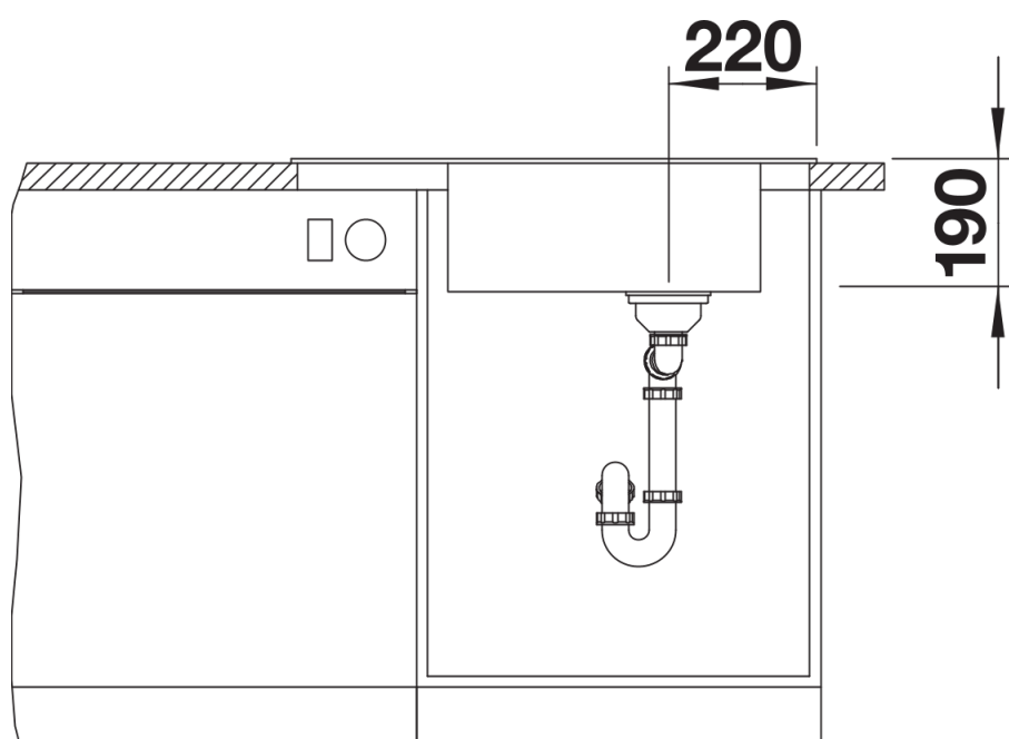
Vista frontale
