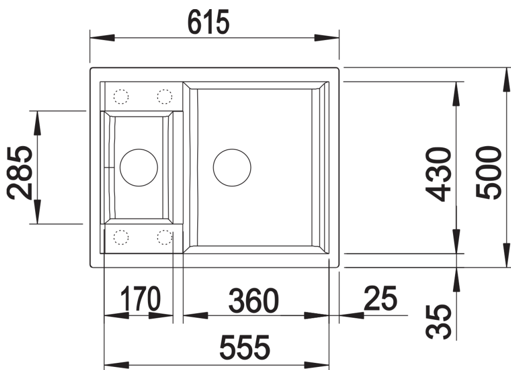
Vista superiore
