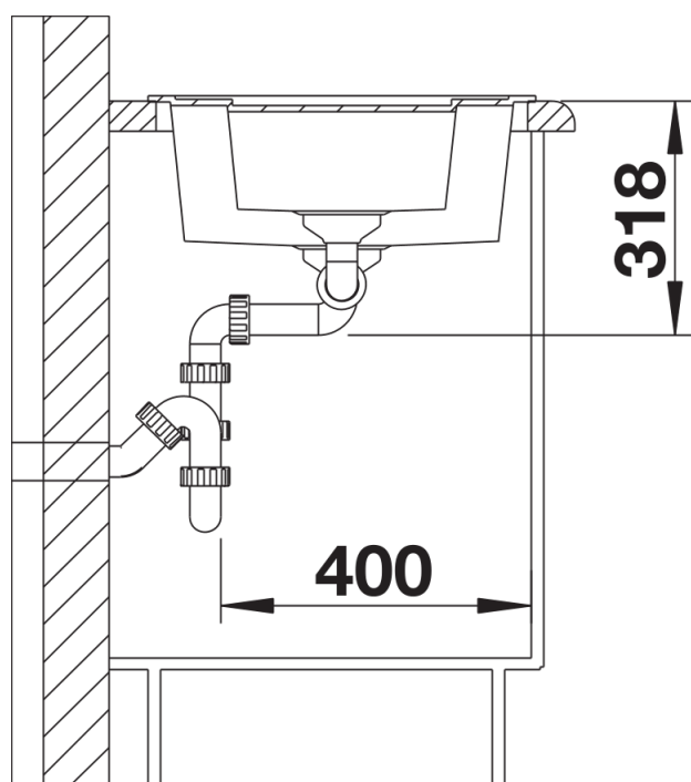
Vista laterale
