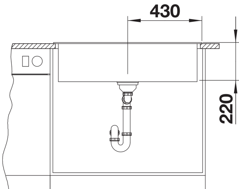
Vista frontale
