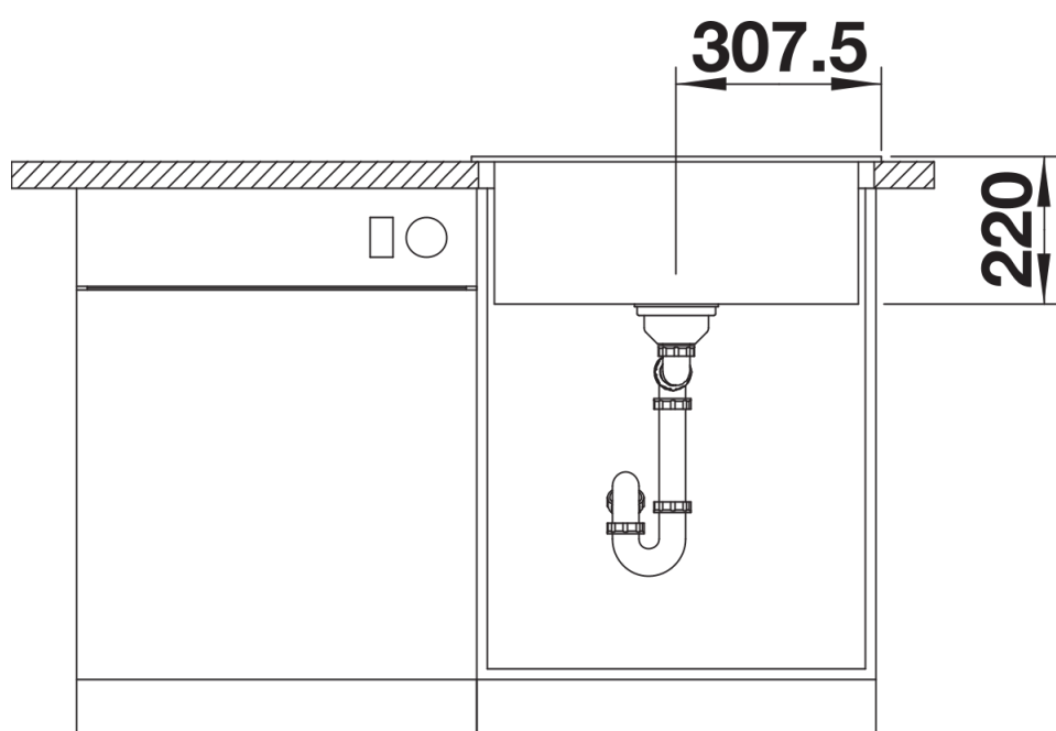
Vista frontale
