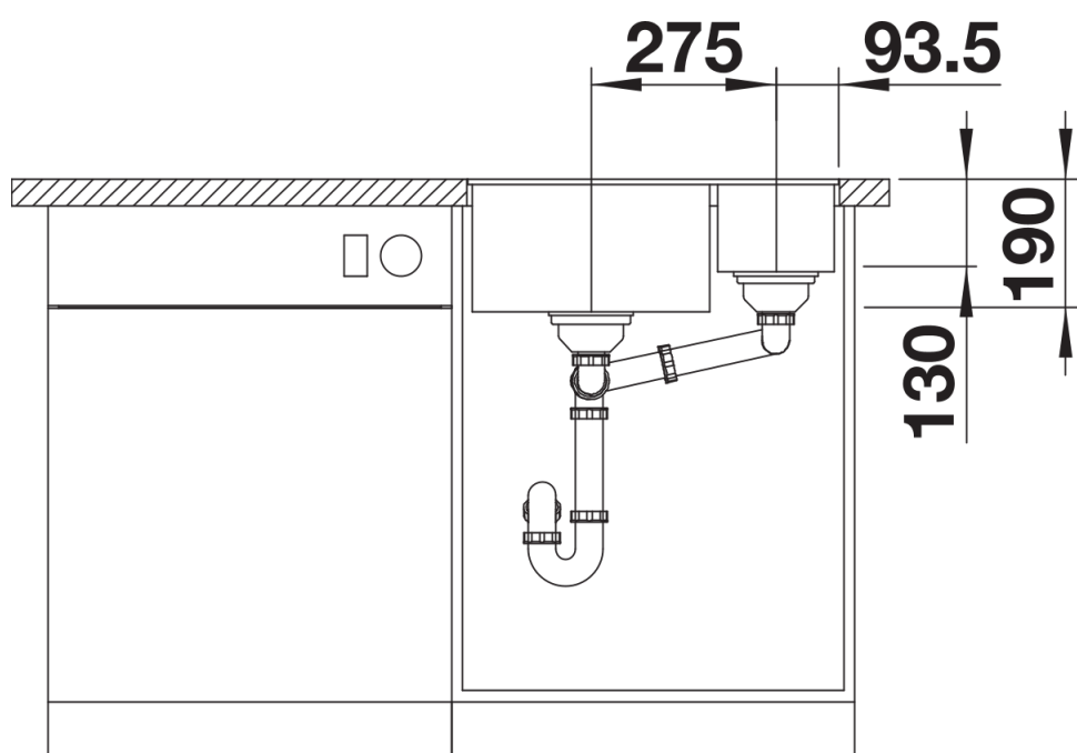
Vista frontale
