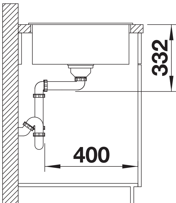
Vista laterale
