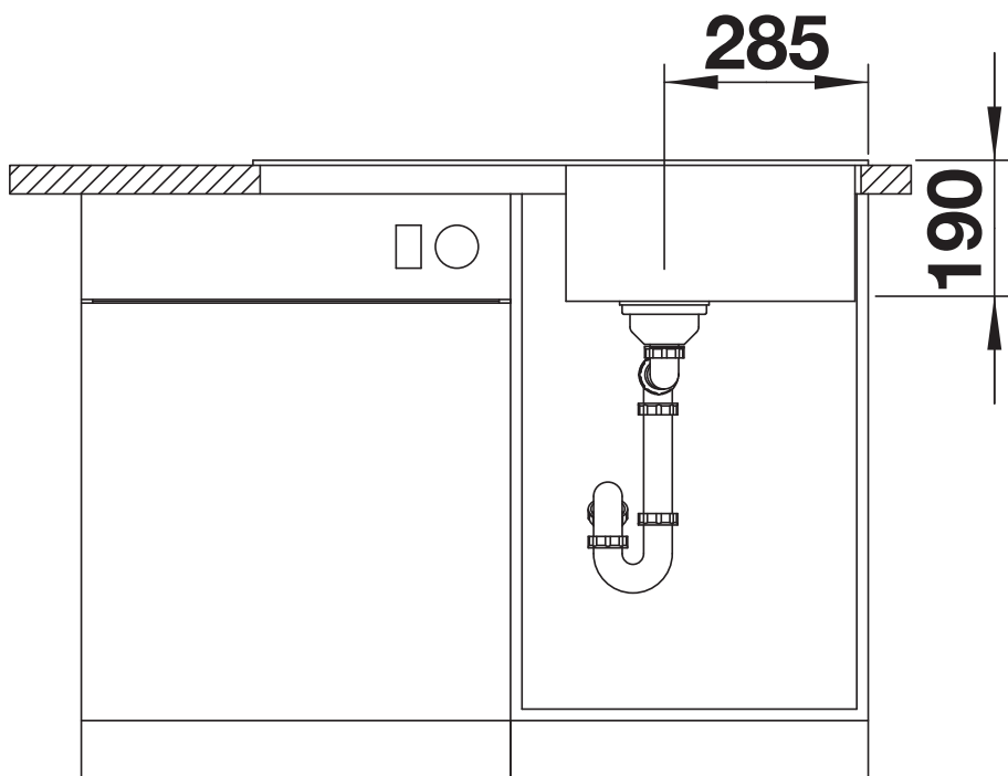
Vista frontale
