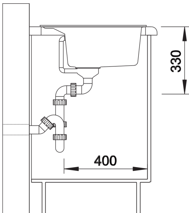
Vista laterale
