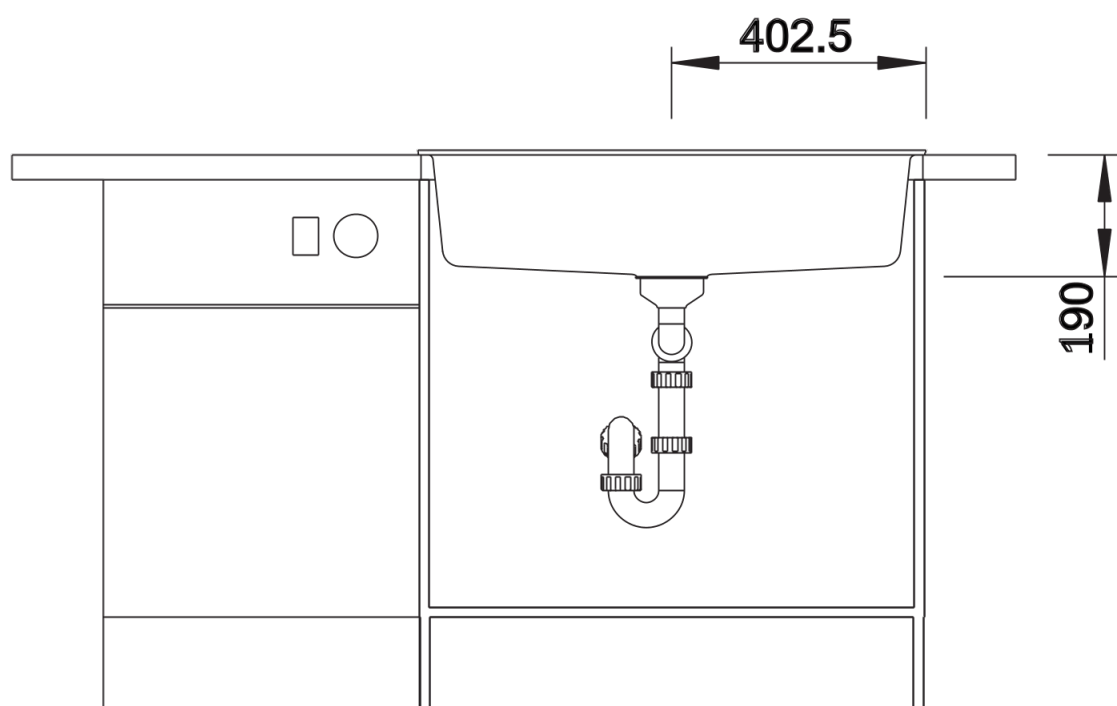
Vista frontale
