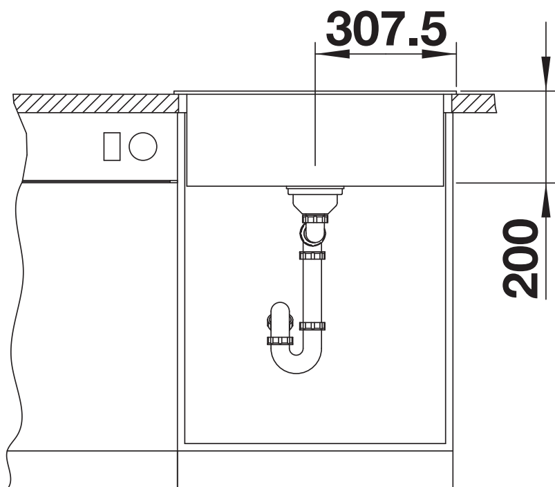
Vista frontale
