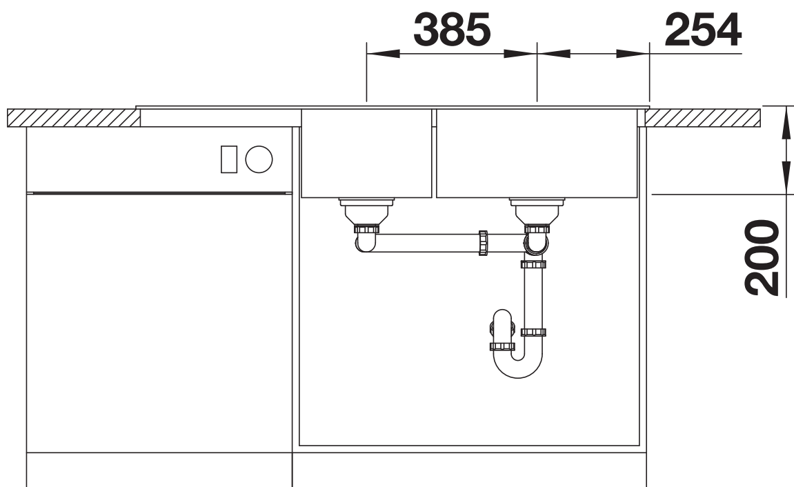
Vista frontale
