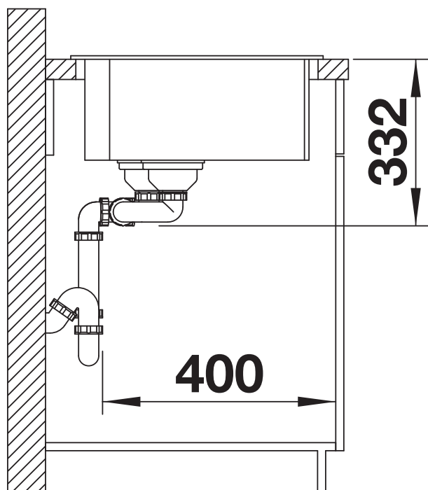
Vista laterale
