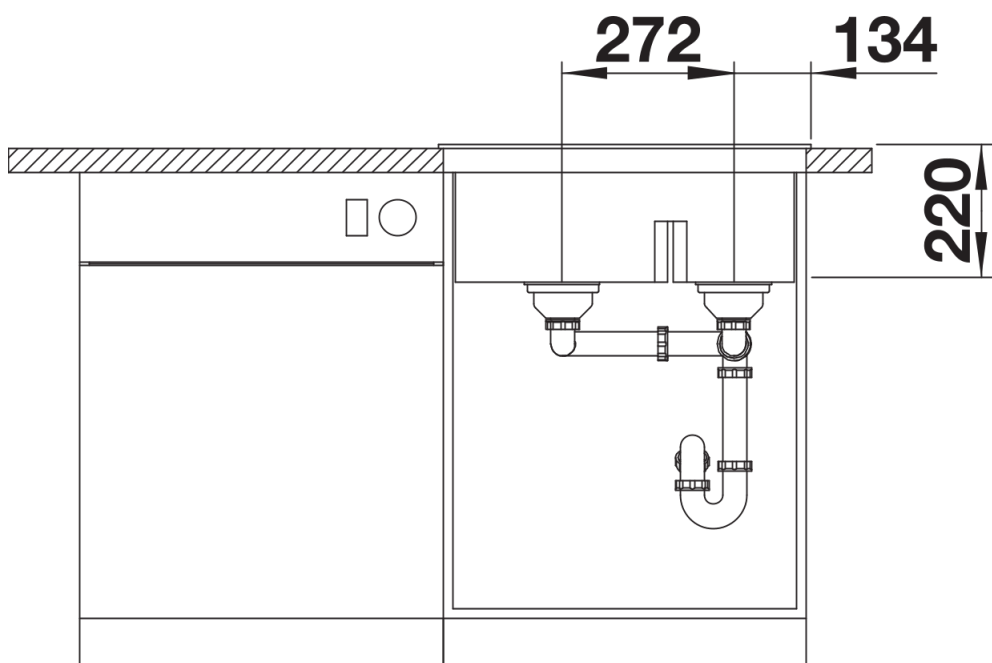
Vista frontale
