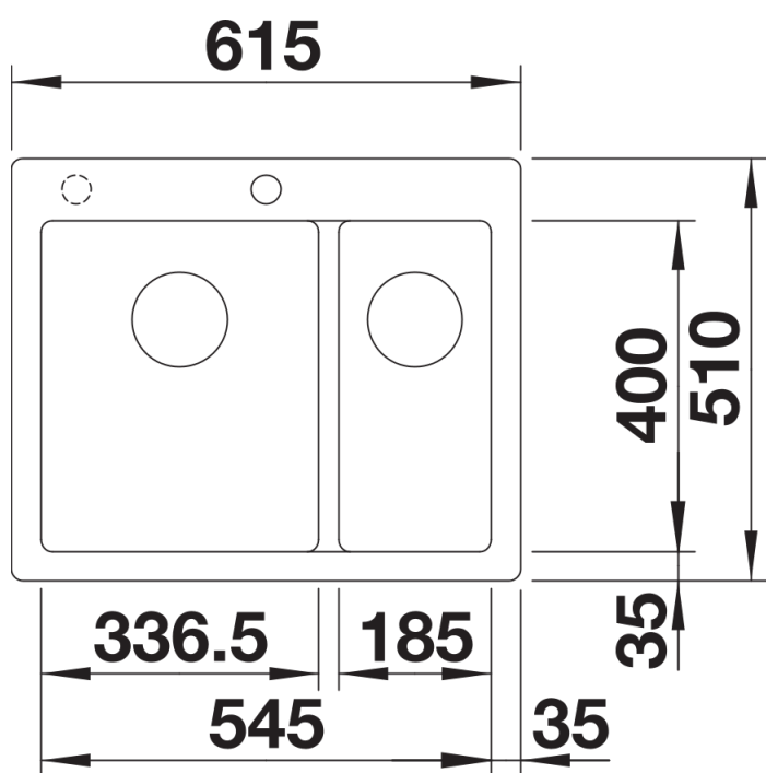
Vista superiore
