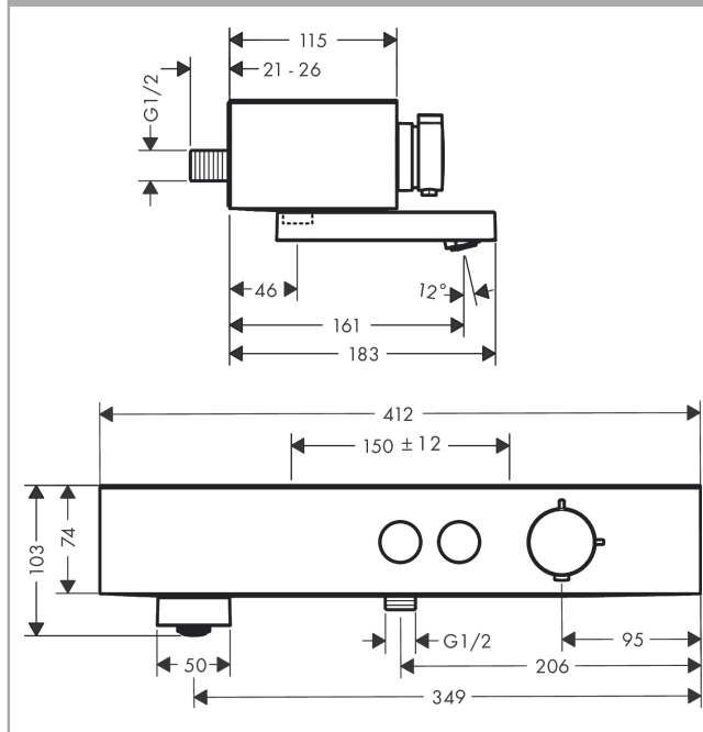
Disegno in scala
